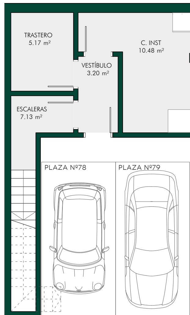
PLANTA SÓTANO
